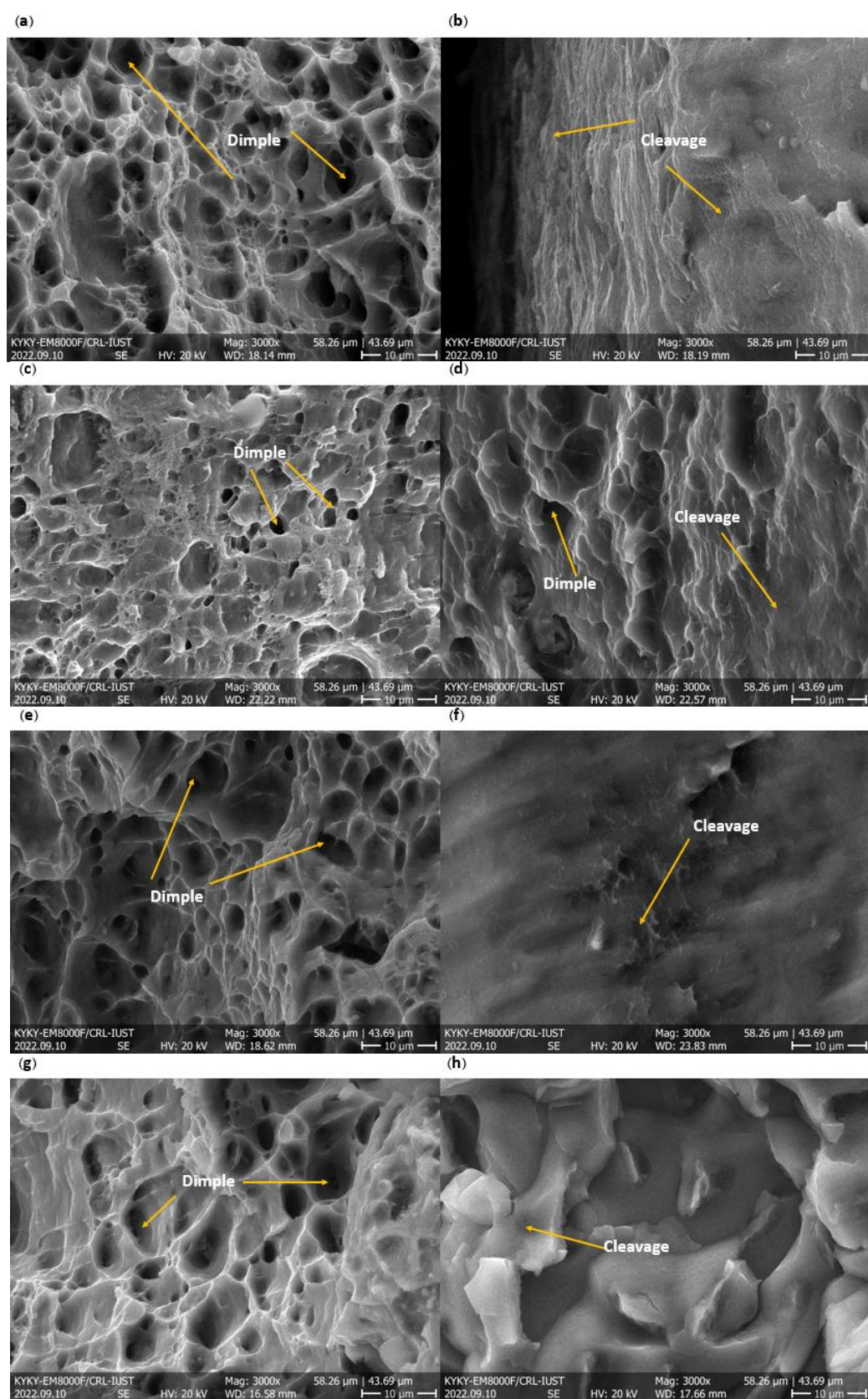
Fig. 14. SEM images from the fracture surfaces, a) 2 -layer Al section- room temperature, b) 2- layer Mg section- room temperature, c) 2- layer Al section-200°C, d) 2- layer Mg section-200°C, e) 2- layer Al section-300°C, f) 2- layer Mg section-300°C, g) 2- layer Al section-400°C, h) 2- layer Mg section-400°C
